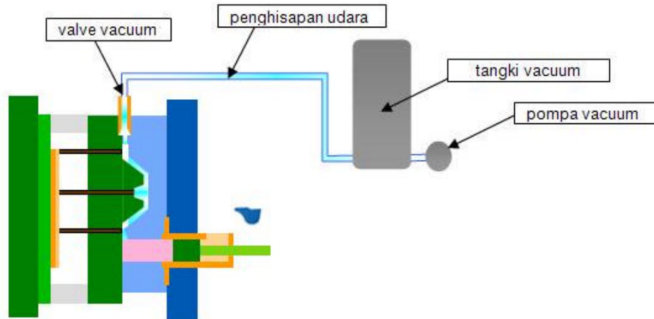
ilustrasi cara kerja dalam metode vacuum casting
